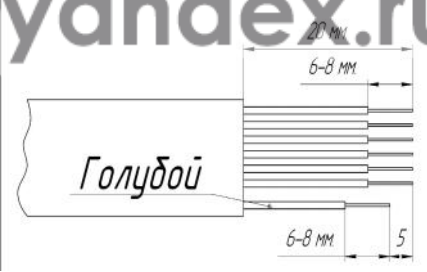
Схема обрезки кабеля
